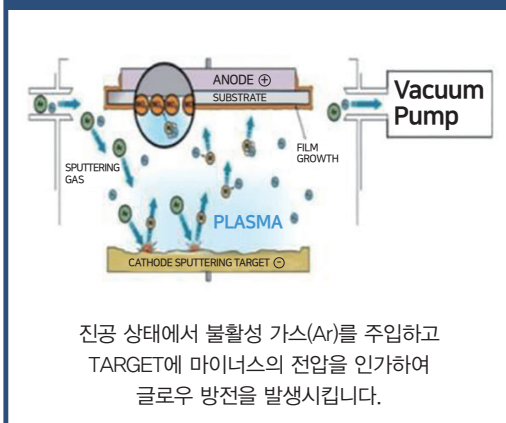
스퍼터의 원리 (1)
